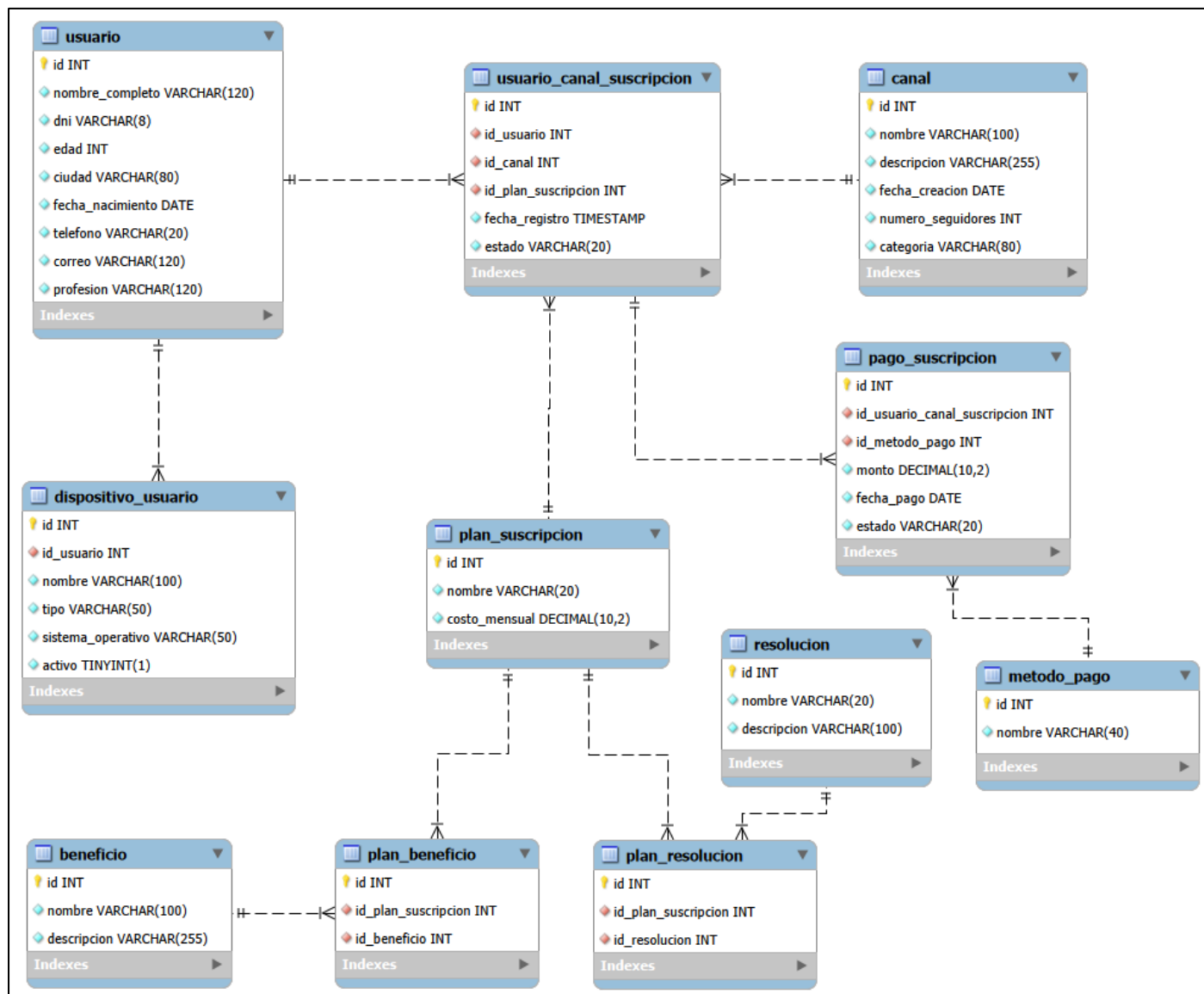
Fig. 01. Diagrama EER de la base de datos para el Caso N° 01: SocialSoft
