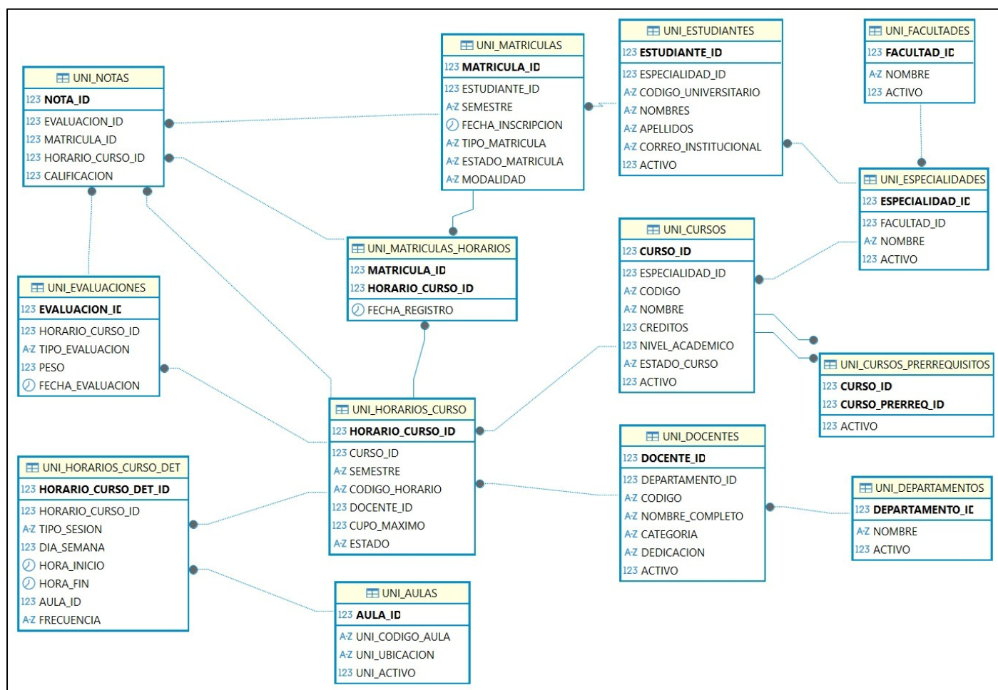
Fig. 02. Diagrama del esquema relacional de la base de datos para el Caso N° 02.
